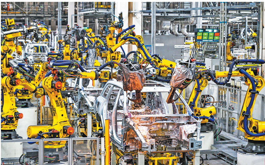
2025年9月19日在位于重庆市两江新区的赛力斯汽车超级工厂拍摄的自动化生产作业现场。
