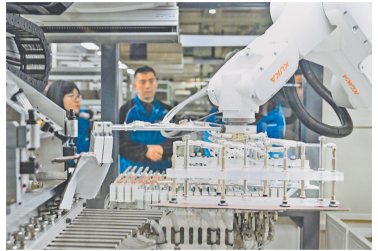
2月18日,位于两江新区的安道拓(重庆)汽车零部件有限公司,黄茅坪工厂机器人缝制工作站正在作业。 记者 张锦辉 摄/视觉重庆
