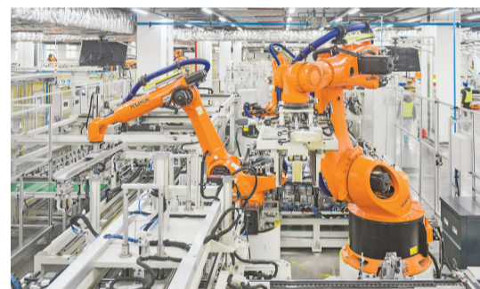
位于龙盛新城的赣锋新型锂电池科技产业园，机械臂在电池PACK产线上自动运行。(摄于1月16日) 记者 张锦辉 摄/视觉重庆
