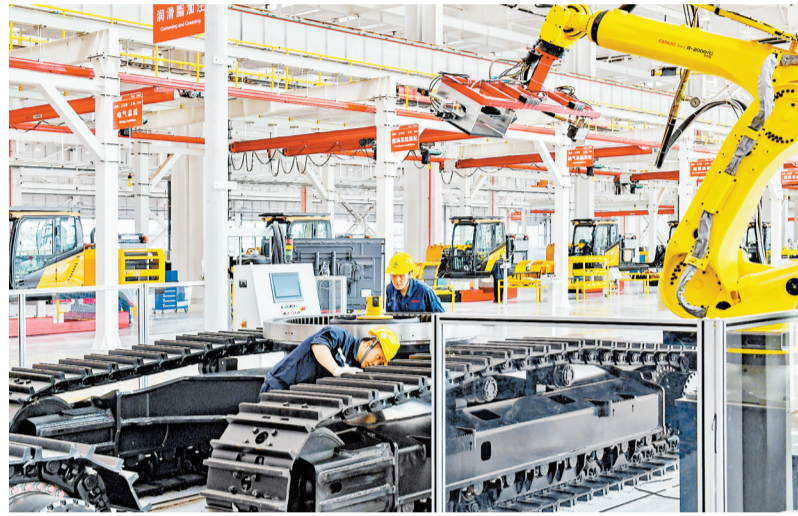
位于两江新区的三一重工生产线,工人正在合车线机器人自动涂胶工位作业。(资料图片) 记者 张锦辉 摄/视觉重庆
