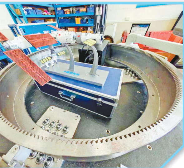
重庆大学机械传动国家重点实验室为问天实验舱配套的对构齿轮传动。(受访者供图)
