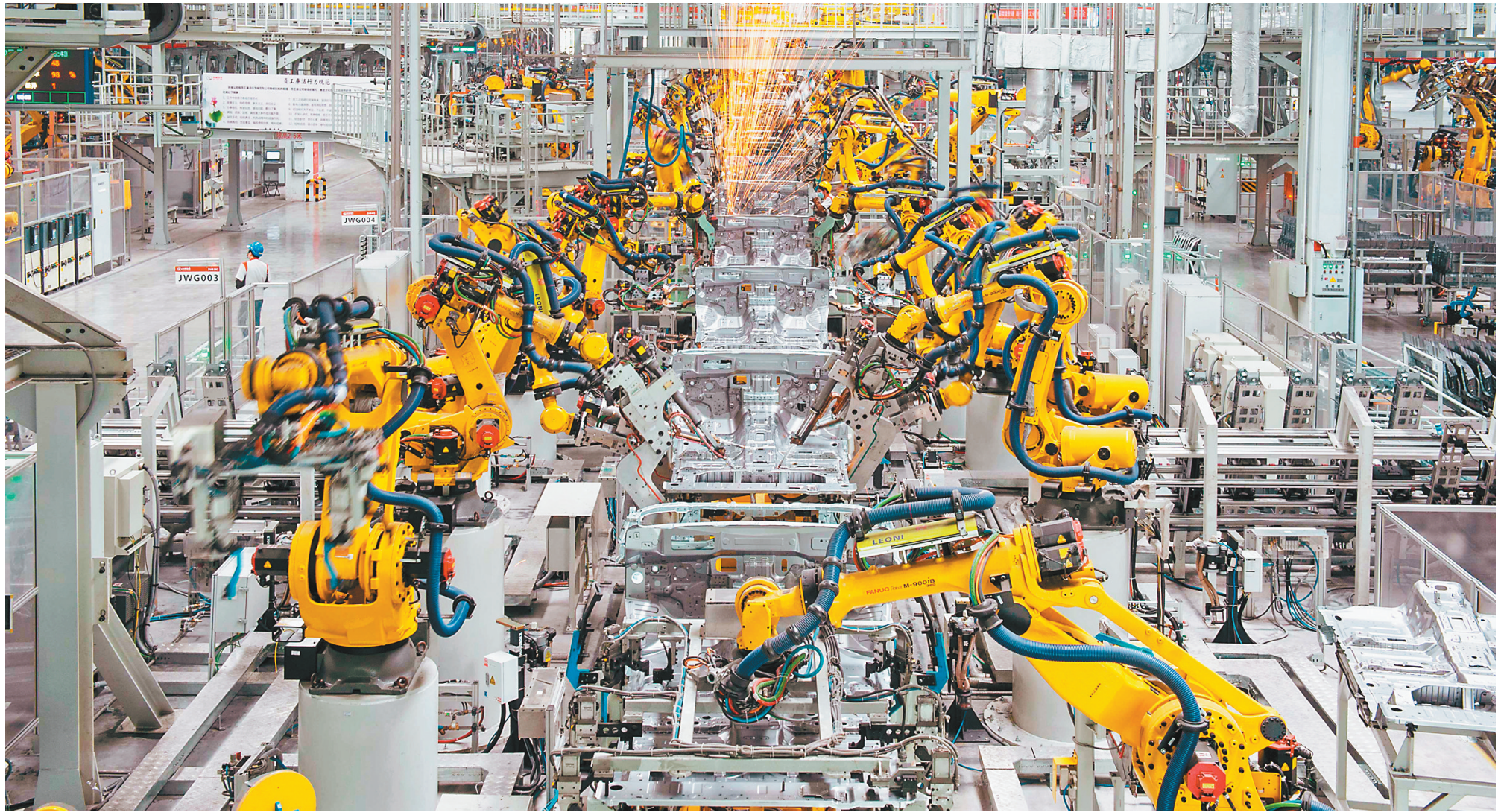
永川长城汽车制造基地内,焊接机器人在工作。(资料图片)
