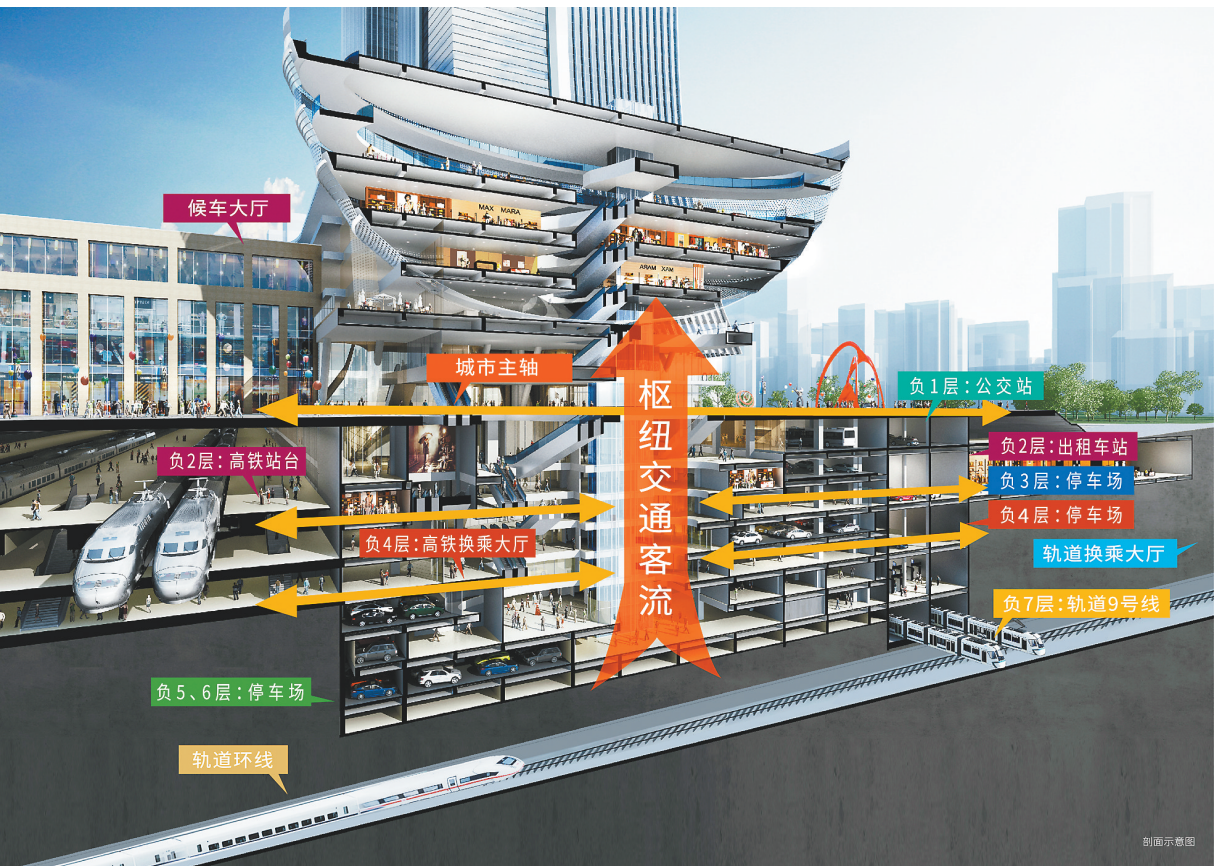
国内首个高速铁路TOD“站城一体化”项目金沙天街剖面示意图。（市规划自然资源局供图）
